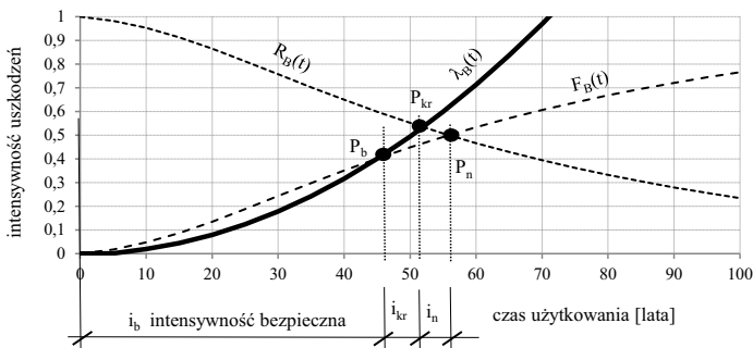
Rys. 1. Zmiany intensywności uszkodzeń w budynku nieremontowanym
