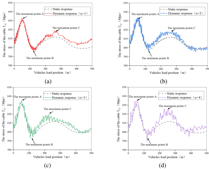
Fig. 18. Stress variation of cable T_{11} : (a) \alpha = 1 ; (b) \alpha = 2 ; (c) \alpha = 3 ; (d) \alpha = 4
